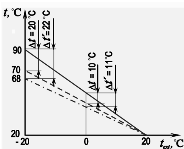
Рисунок 7.9 – Определение требуемого перепада теплоносителя в отопительном приборе.
