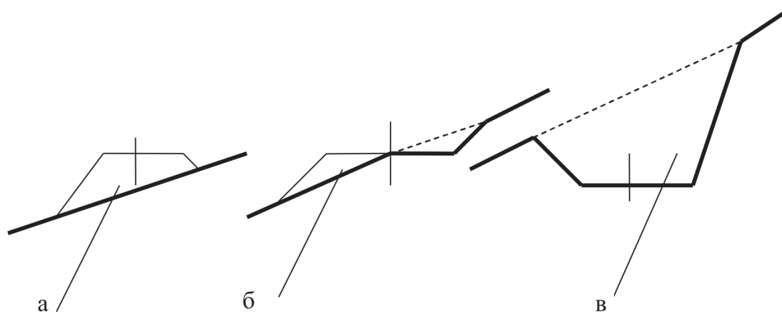
а) насыпь; б) полунасыпь-полувыемка; в) выемка
