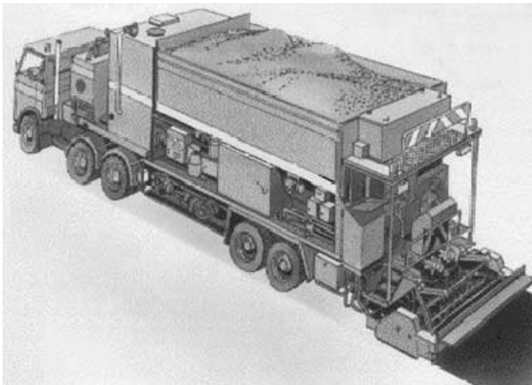
Рисунок С.2 – Общий вид машины для устройства литой эмульсионно-минеральной смеси
